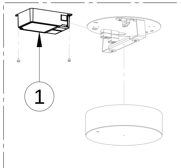
DETTAGLIO A
