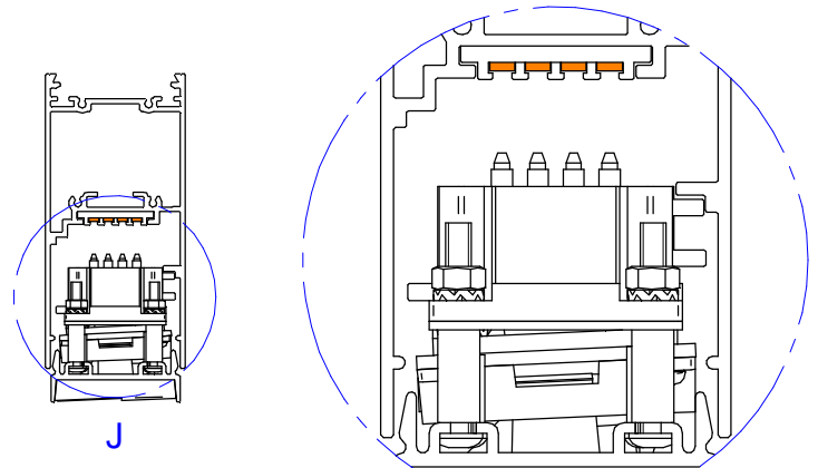
DETTAGLIO J
