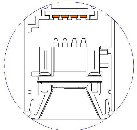
DETTAGLIO B
