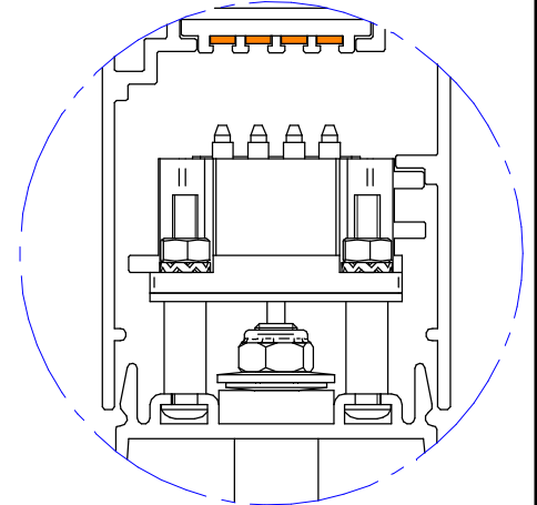
DETTAGLIO H
