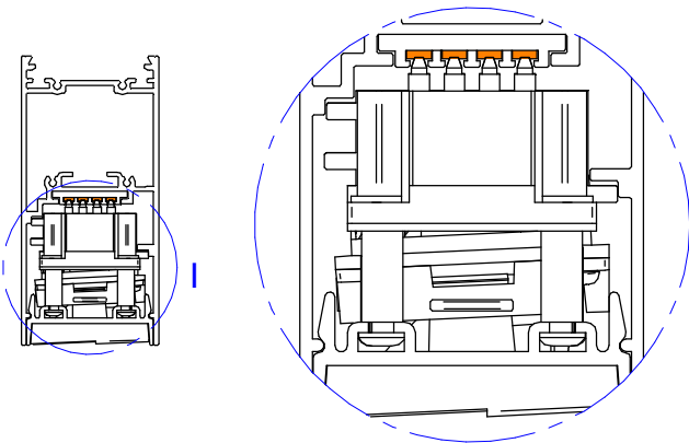
DETTAGLIO I
