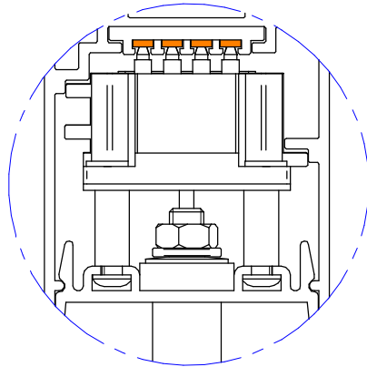
DETTAGLIO G
