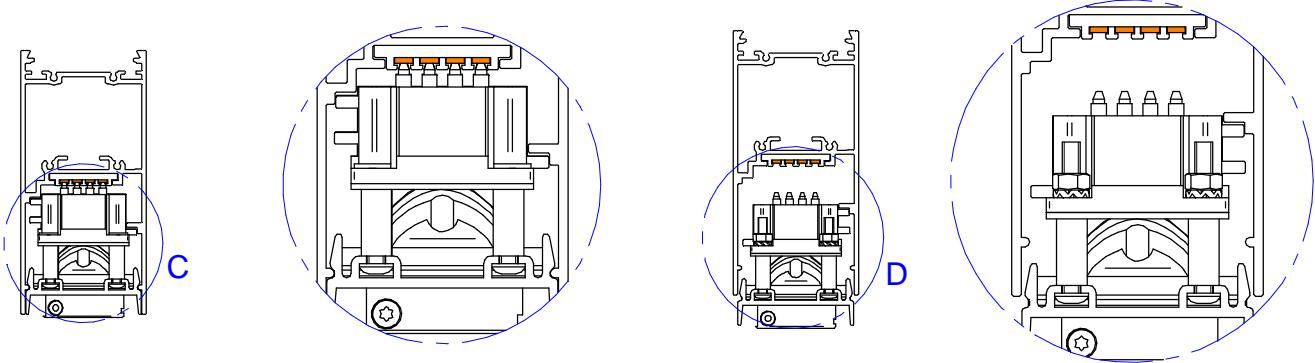
DETTAGLIO C
