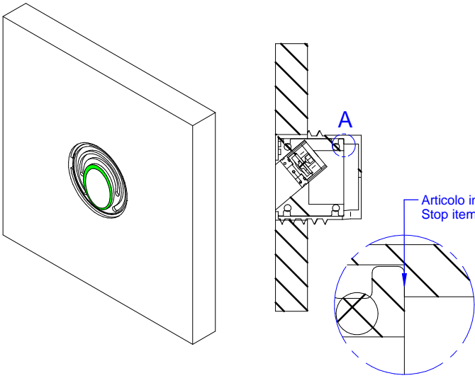
DETTAGLIO A
