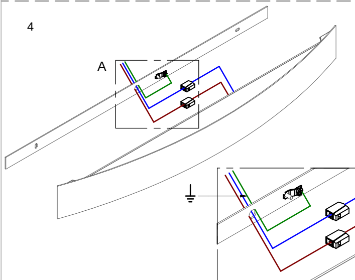
DETTAGLIO A
