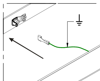
DETTAGLIO B
