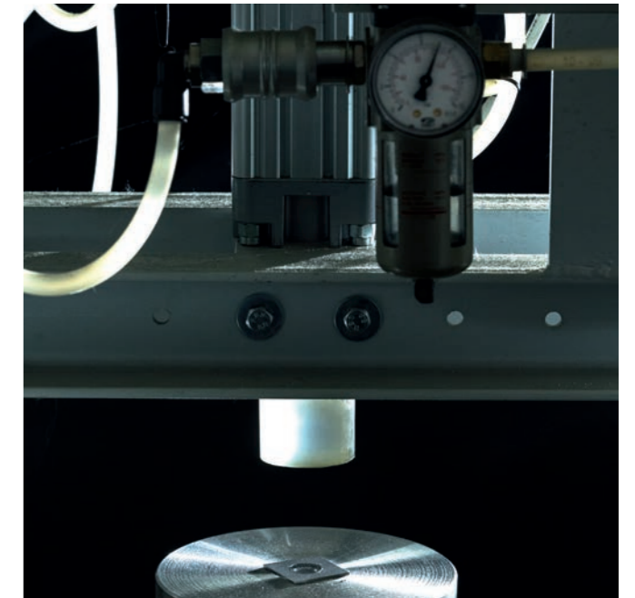
Test IK IK test
